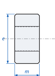
Trapezoidal Thread Hex Nut DIN 103 - dimensions
