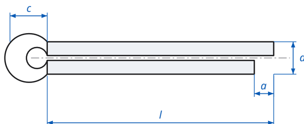
Split Cotter Pin DIN 94 / ISO 1234 - dimensions
