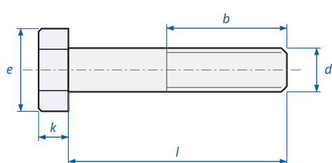
Structural Hex Bolt EN 14399 - dimensions
