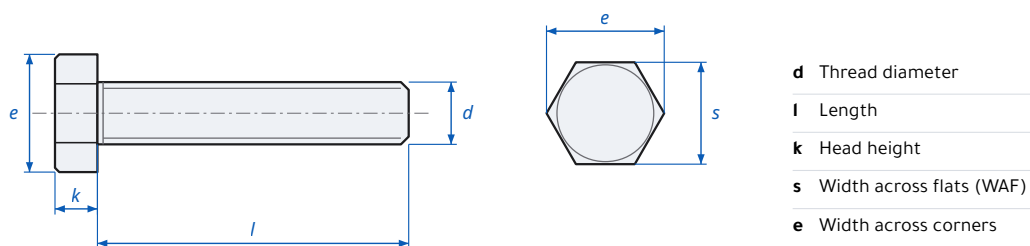
Hex Head Screw DIN 933 / ISO 4017 - dimensions
