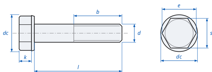
Hex Flange Bolt DIN 6921 - dimensions
