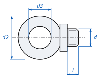
Eye Bolt Form B DIN 444B - dimensions
