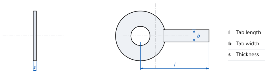
Tab Washer with Long Tab DIN 93 - dimensions
