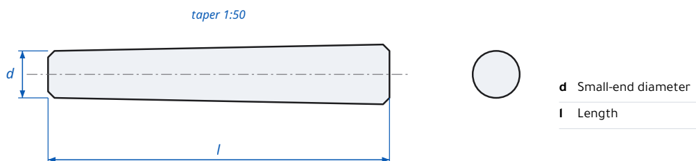
Taper Pin DIN 1 - dimensions
