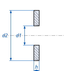
Flat Washer DIN 125A / ISO 7089 - dimensions
