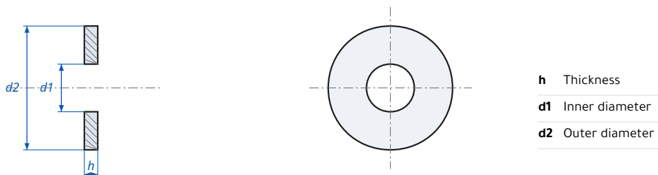
HV Structural Washer DIN 6916 / EN 14399-6 - dimensions
