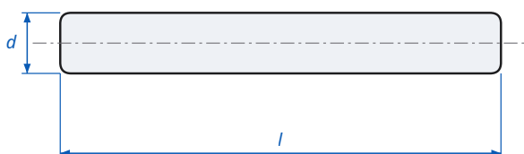
Parallel Pin DIN 7 / ISO 2338 - dimensions
