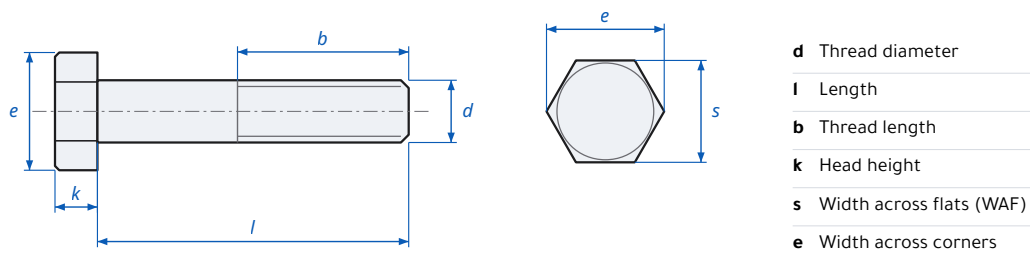
Hex Head Bolt DIN 931 / ISO 4014 - dimensions
