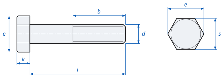
HV Structural Hex Bolt DIN 6914 / EN 14399-4 - dimensions
