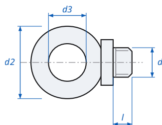
Eye Bolt Form A DIN 444A - dimensions
