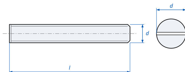
Slotted Set Screw Flat Point DIN 551 - dimensions
