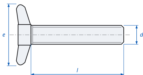
Wing Screw DIN 316 - dimensions
