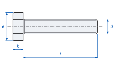
Hex Head Screw DIN 933 / ISO 4017 - dimensions
