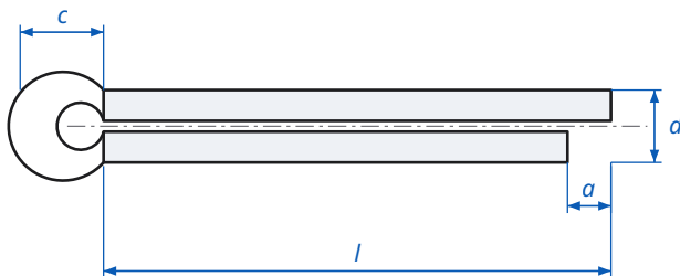
Split Cotter Pin DIN 94 / ISO 1234 - dimensions
