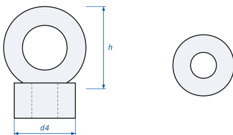
Lifting Eye Nut DIN 582 - dimensions
