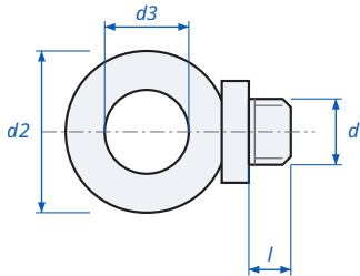
Eye Bolt Form B DIN 444B - dimensions
