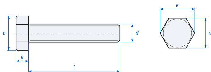
Hex Head Screw DIN 933 / ISO 4017 - dimensions
