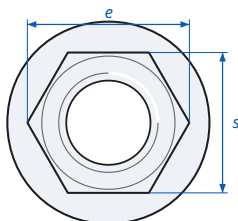
All-Metal Hex Flange Lock Nut DIN 6927 - dimensions
