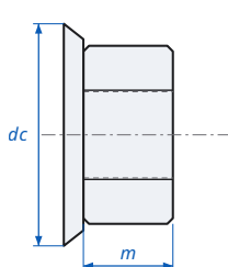
All-Metal Hex Flange Lock Nut DIN 6927 - dimensions
